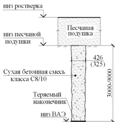
Рис. 1 – Схема геомассива
